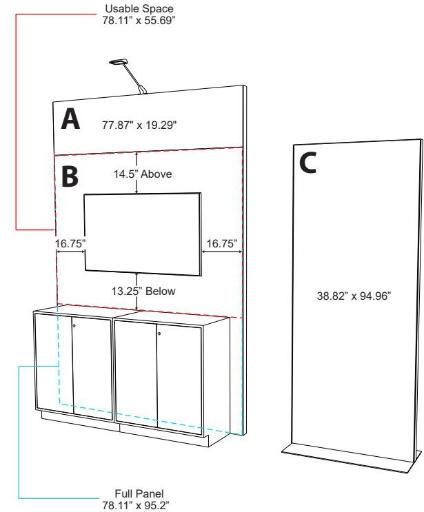
OPTION 3 Optional 55" Monitor
